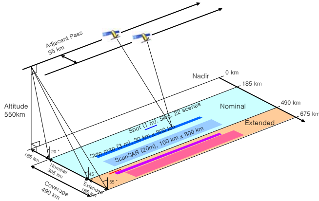
Fig. 1. Imaging modes of KOMPSAT-5 SAR.
