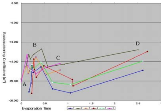
그림 2. Radarsat-1 SAR 조건대 영상에서 증발시간에 따른 후방산란계수.
